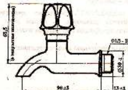
Рисунок 1. Кран КрН15
